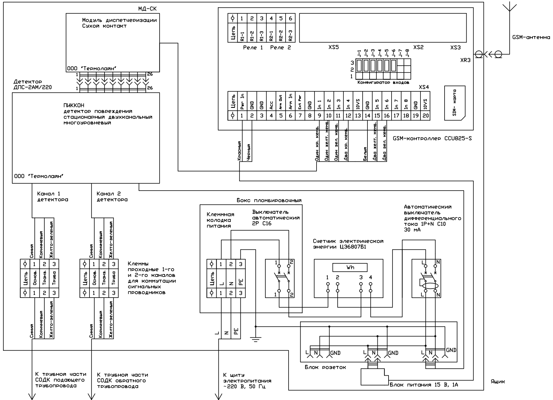
Электрическая схема подключений комплекта оборудования ДПС-220/СК
